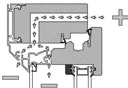
Övertryck i rummet gör att luften pressas ut genom ventilen och vidare ner mellan bågarna och ut.
